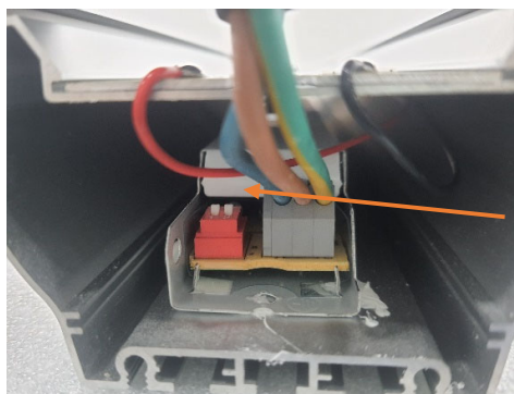
Nút gạt điều chỉnh 4 cấp công suất
